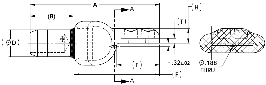
SECTION A-A SCALE 1 : 3
